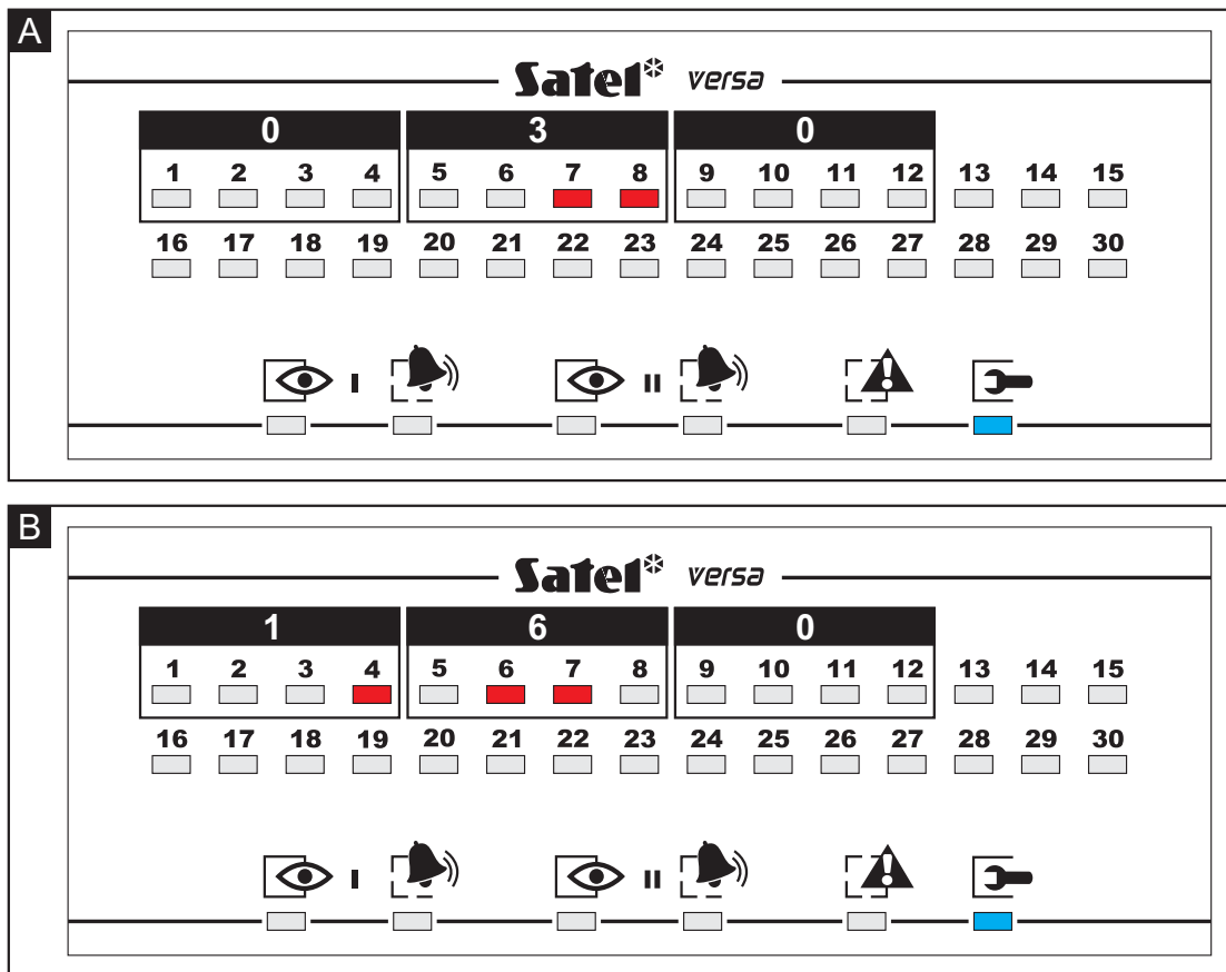
Rys. 1. Przykłady prezentowania wartości dziesiętnych przy pomocy diod LED w manipulatorze VERSA-LED-GR. W przykładzie A zaprogramowana jest wartość 30 (030), a w przykładzie B – 160.
