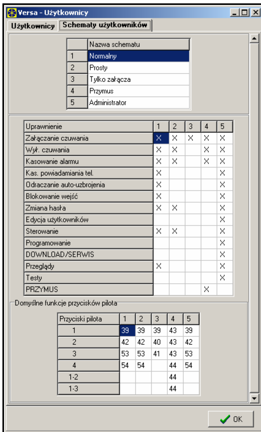
Rys. 19. Programowanie schematów użytkowników w oknie „Versa – Użytkownicy” w programie DLOADX (przykładowe ustawienia).
